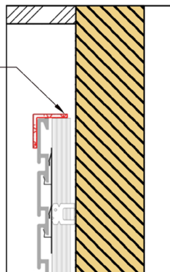
Вид сбоку
