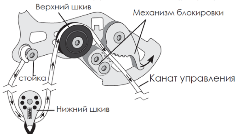
Рис. 2: Самоблокирующаяся скоба (разрез)
