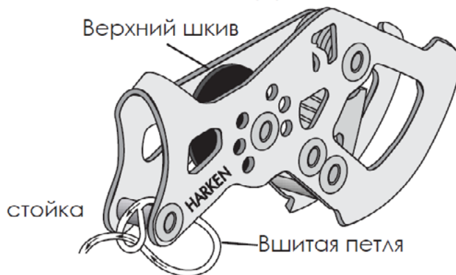
Рис. 1: Самоблокирующаяся скоба
